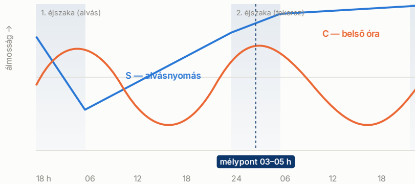
1. ábra · A két-folyamat modell sémája 48 órán át egy átalvott és egy áttekert éjszakával. Sematikus rajz, nem mért görbe. Forrás: Borbély-modell A
